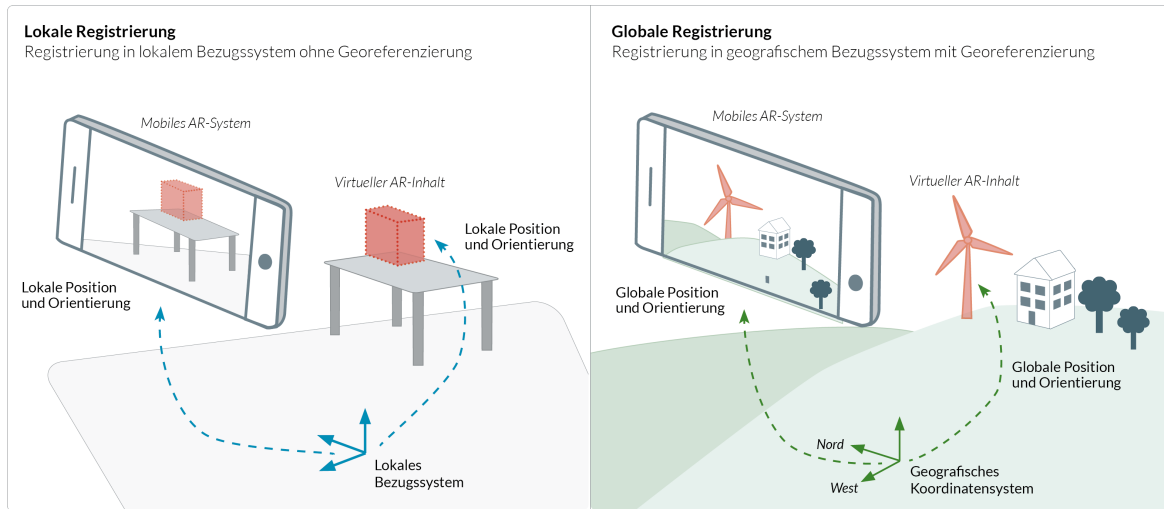
Abbildung 2.2 Bei der lokalen Registrierung werden das AR-System sowie die virtuellen AR-Inhalte in Bezug auf ein lokales Bezugssystem ohne Georeferenzierung definiert (links). Bei der globalen Registrierung sind virtuelle AR-Inhalte in Bezug auf ein globales geografisches Bezugssystem definiert (rechts). Eine Georeferenzierung der Geräte-Pose des mobilen AR-Systems ist dann notwendig.
