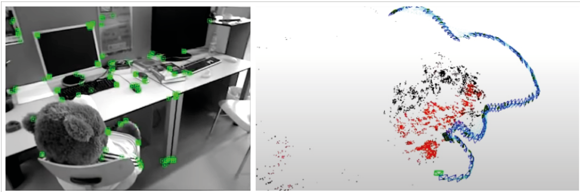
Abbildung 3.3 Registrierung in unbekannter Umgebung mittels monokularer SLAM-Technologie, z.B. ORB-SLAM [102]. In den Kamerabildern werden markante Feature-Punkte der Umgebung erfasst (links; grüne Punkte) und in einer 3D-Punktwolken-Karte gespeichert (rechts; rote Punkte). Mit zunehmender Kamerabewegung kann die Karte erweitert und die Kamerapositionen innerhalb dieser Karte fortlaufend erfasst werden (rechts; blauer Pfad).
