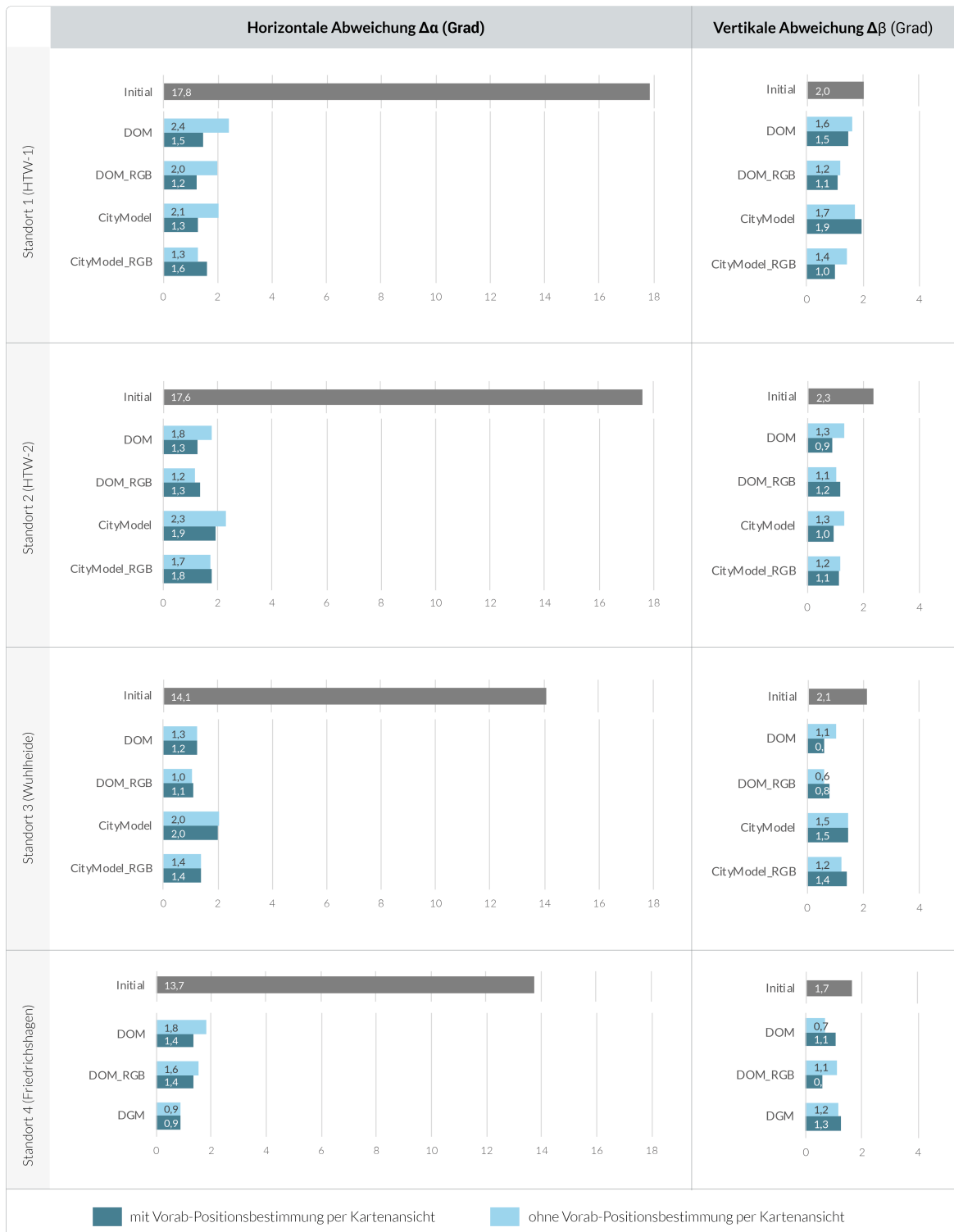
Abbildung 5.11 Gemessene durchschnittliche horizontale und vertikale Abweichung der kalibrierten globalen Gerätorotation.
