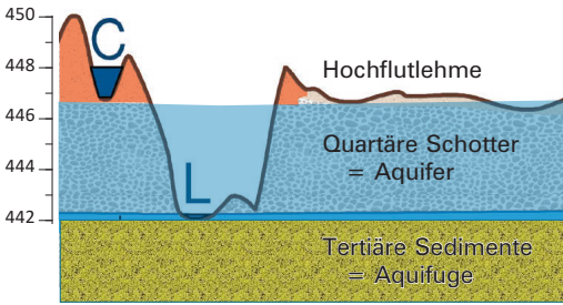
Abb. 3. Topografischer Schnitt durch die Lechauen in Höhe von Gersthofen, mit Lech (L) und Lechkanal (C). Die Grundwasseroberfläche wurde von knapp 447 m auf mittlerweile 442 m abgesenkt. Braun gefärbt: technische Substrate; kräftig blau: jetziger Grundwasserstand; durchscheinend blau: ursprünglicher Grundwasserstand vor den Lech-Correctionen. – Topographie aus BayernAtlas-plus , Bayerisches Landesamt für Vermessung; Fluss- und Grundwasserspiegel vom Niedrigwasser-Informationsdienst, www.nid.bayern.de .
