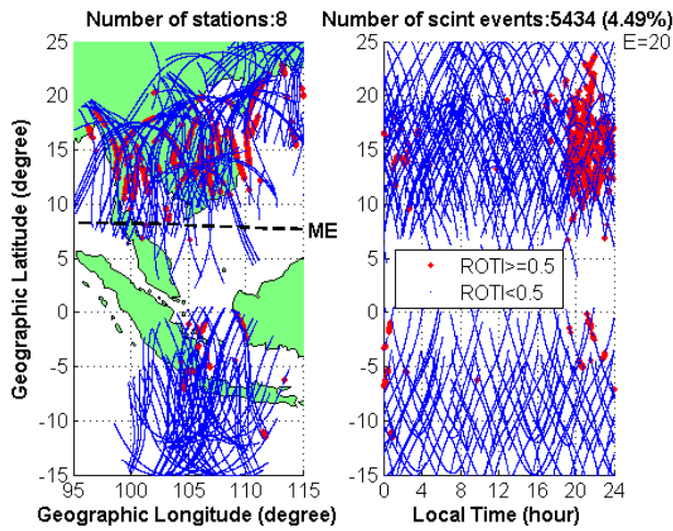
d1. Regional ROTI map on 31 st
