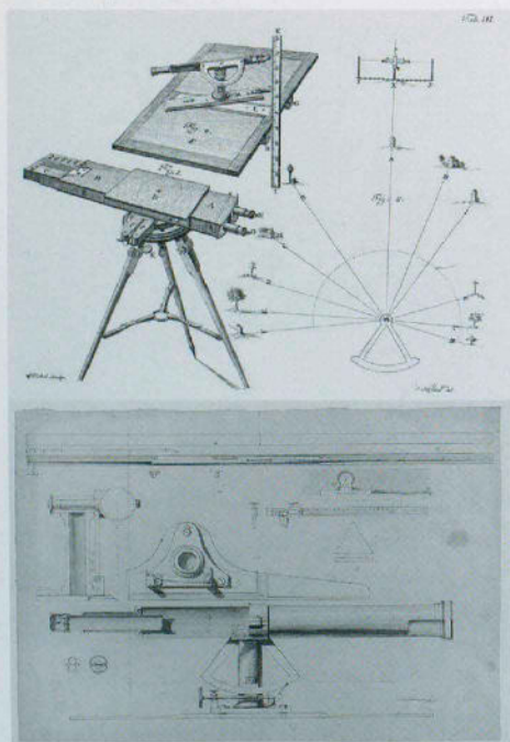
Oben: Entfernungsmessung mit Kippregel nach Brander, Kupferstich von 1767.
