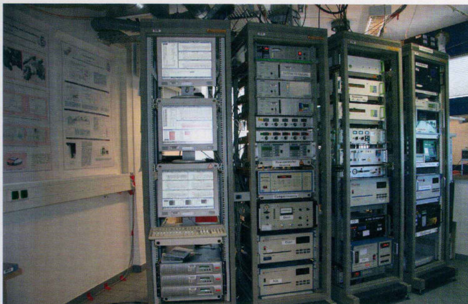
Luftchemische Messgeräte, mit denen ab 1995 die Veränderung der Spurenstoffe der Luft im Rahmen des Global Atmosphere Watch Programms der World Meteorological Organisation überwacht wird.
