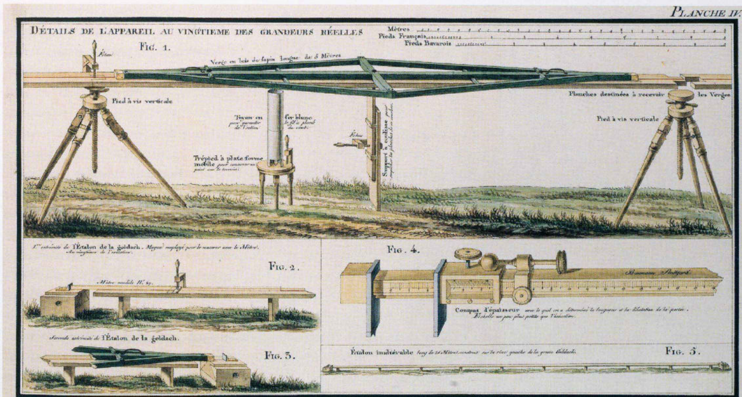
Plan [Planche IV] einer 5 Meter langen Messstange von Oberst Bonne. Aquarell von Daumiller, ca. 1806/08.
