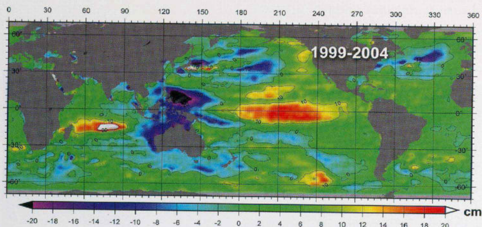
Aktueller Forschungsschwerpunkt des DGFI ist die Messung und Analyse globaler Veränderungen. Im Bild ist der Meeresspiegelanstieg von 1999 bis 2004 dargestellt, der im globalen Mittel 3,4 mm/Jahr beträgt.
