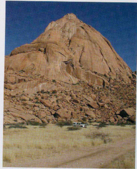
Der Inselberg „Spitzkoppe“ auf der Haupttrumpffläche in Namibia.
