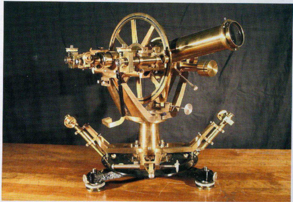
Astronomisches Universal von A. Repsold u. Söhne, Hamburg 1893.
