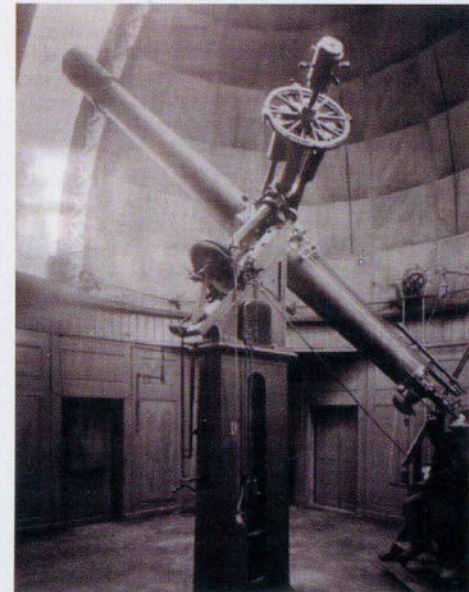
Der 1835 aufgestellte Fraunhofer'sche Refraktor war seinerzeit mit seinem Objektivdurchmesser von 28,5 cm und der Güte seiner Optik für vier Jahre das beste Teleskop der Welt. Der Auftrag zum Bau war Fraunhofer schon 1825 erteilt worden. Er hatte noch vor seinem Tod 1826 die Montierung des Teleskops konzipiert und den Glasblock geschmolzen, aus dem später sein Nachfolger Georg Merz (1793–1870) das Objektiv schliiff. Die Aufnahme entstand um 1900.
