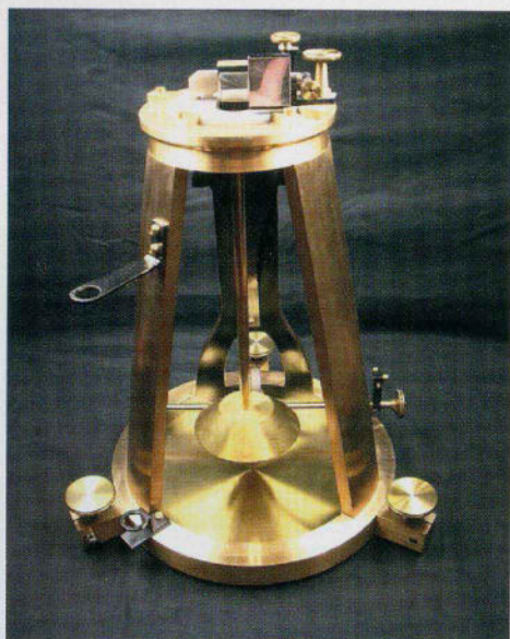
Pendelapparat von E. Schneider, Wien 1896.
