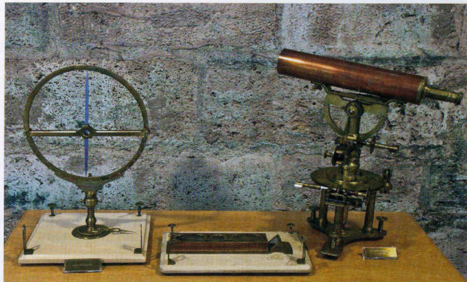
Inklinatorium und Deklinatorium zur Messung der Vertikal- und Horizontalkomponente des Erdmagnetfeldes. Rechts das Observatorium portabile, ein Fernrohr mit Winkelmesseinrichtung. Alle Geräte wurden von Brander in Augsburg vor 1780 gebaut.
