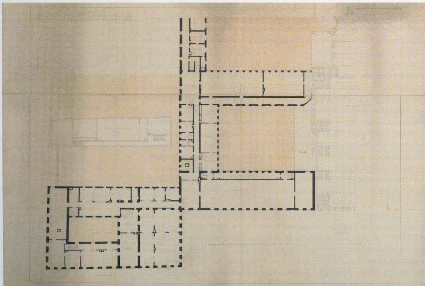
Grundrissplan der so genannten „Alten Akademie“, dem ehemaligen Jesuitenkolleg (Wilhelminum) in der Neuhauser Straße in München, 1784/1844. Von 1783 bis 1843 war die Hofbibliothek hier untergebracht.
