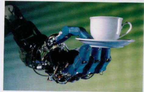
Künstliche 4-Finger-Hand mit 12 Bewegungsfreiheitsgraden samt Leichtbauroboter mit 7 Bewegungsfreiheitsgraden.
