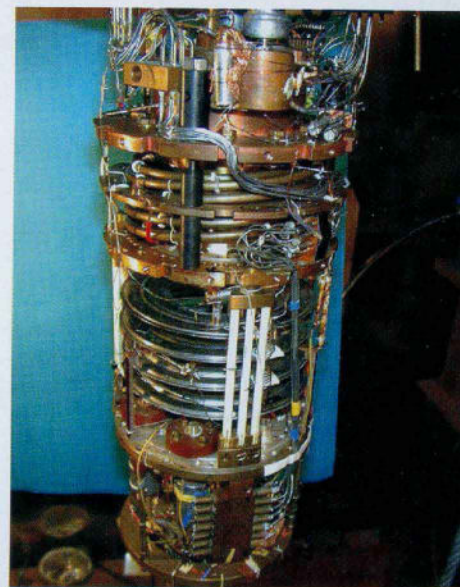
Mischkühler-Einheit des Kernentmagnetisierungskryostaten „Millimühle 2“ des Walther-Meißner-Instituts.
