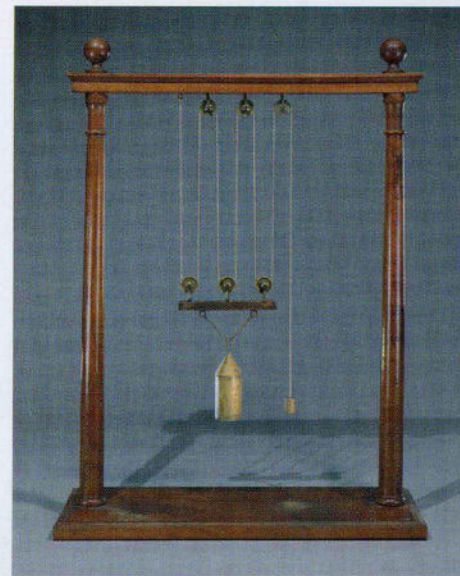
Flaschenzug in der Sammlung der Bayerischen Akademie der Wissenschaften (18. Jahrhundert). Der Flaschenzug und seine Funktionsweise waren im 18. Jahrhundert ein wichtiges Thema in Vorlesungen zur Mechanik.
