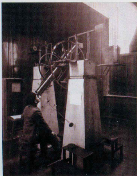
Der Meridiankreis von Reichenbach und Ertel nach einer Photographie, die um 1900 entstand. Er war bei seiner Lieferung 1819 einer der besten Meridiankreise der Welt, da seine Kreisteilung mit Reichenbachs berühmter Kreisteilmachine vorgenommen worden war, die eine Verbesserung der Deklinationsbestimmung von Sternen um einen Faktor 10 brachte.
