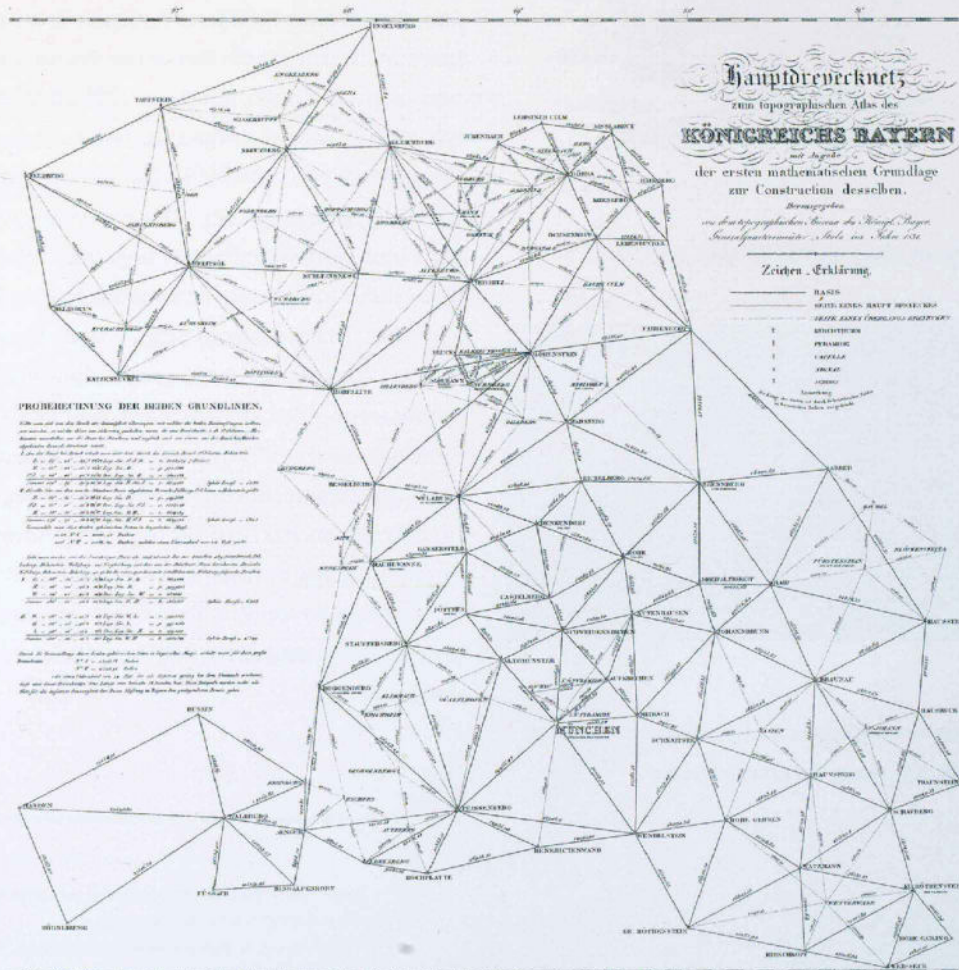
Hauptdreiecknetz zum Topographischen Atlas von 1831.
