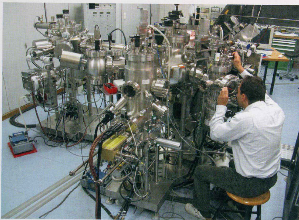
Ultrahochvakuum-System zur Herstellung und Charakterisierung dünner magnetischer oder supraleitender Schichten.
