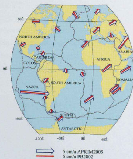
Das Bild zeigt die Erdkrustenbewegungen aus geophysikalischen Beobachtungen über 3 Millionen Jahre (PB2002) im Vergleich mit Bewegungen der letzten 25 Jahre (APKIM2005).
