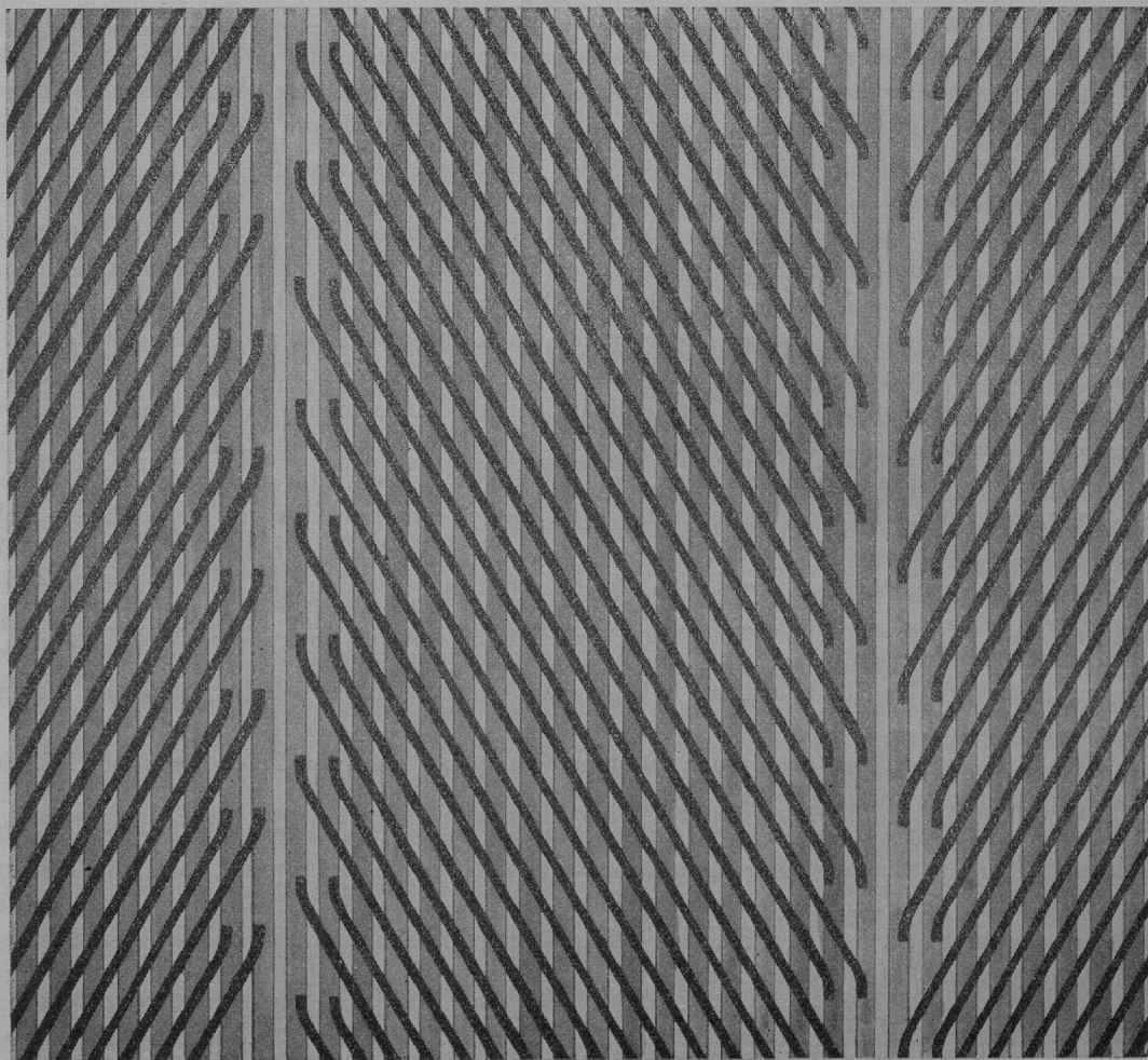
Schema des Verlaufes der eigentlichen Blattspurbündel (grau) und der Nebenbündel (schwarz) eines Blattspurbündelkreises. Das Schema ist so gezeichnet, daß man auf einen an einer Stelle längs geöffneten und planausgebreiteten Blattspurbündelkreis vom Stamminnern aus hinblickt. In der Mitte der rechten Hälfte der Figur die Stelle der Nebenbündelabgabe, in der Mitte der linken Hälfte der Figur die um 180^\circ gegenüberliegende Stelle der Nebenbündelaufnahme.
