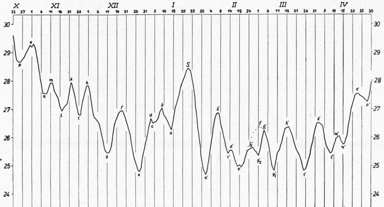
Bild 8. Verlauf des Luftdrucks auf der Zugspitze (500 + .. mm) im Winterhalbjahr in übergreifenden Pentadenmitteln für die Jahre 1901-1930
