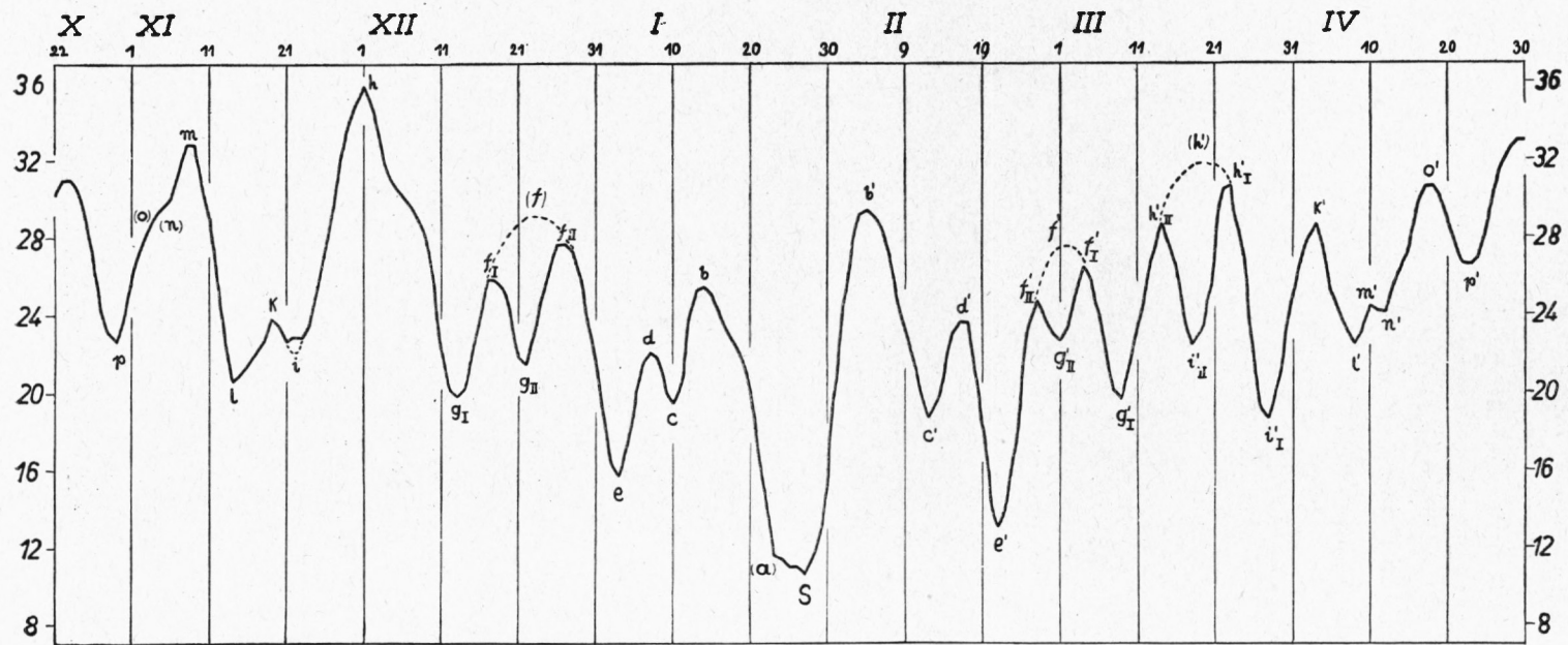
Bild 23. Gang des Luftdrucks auf der Zugspitze in übergreifenden Pentadenmitteln (500 + .. mm) im Winter 1914/15
