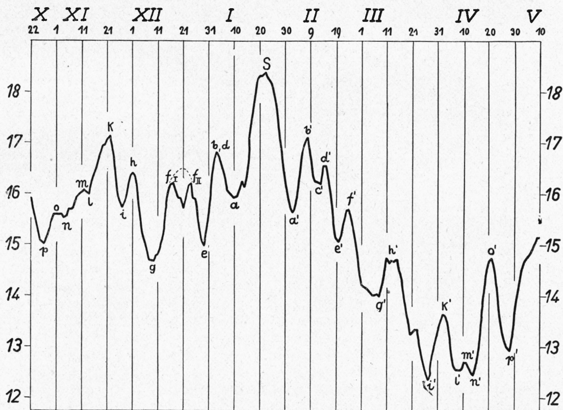
Bild 11. Verlauf des Luftdruckes in München im Bereiche des Winterspiegelungspunktes in übergreifenden Pentadenmitteln
