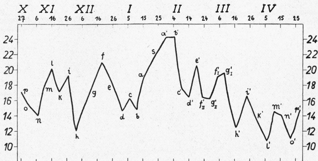
Bild 19. Mittlere Abweichungen des Luftdrucks in mm an den markanten Punkten der einzelnen Jahre im Winterabschnitt
