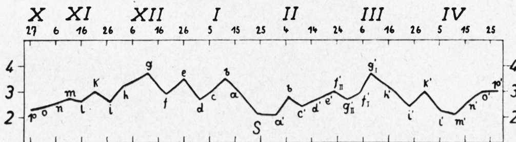
Bild 15 Mittlere Streuung des Eintrittsdatums der markanten Punkte im Winter
