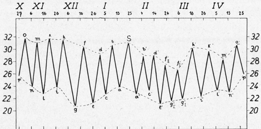
Bild 17. Mittlere Luftdrucke an den markanten Punkten des Winterhalbjahrs (500 + .. mm)
