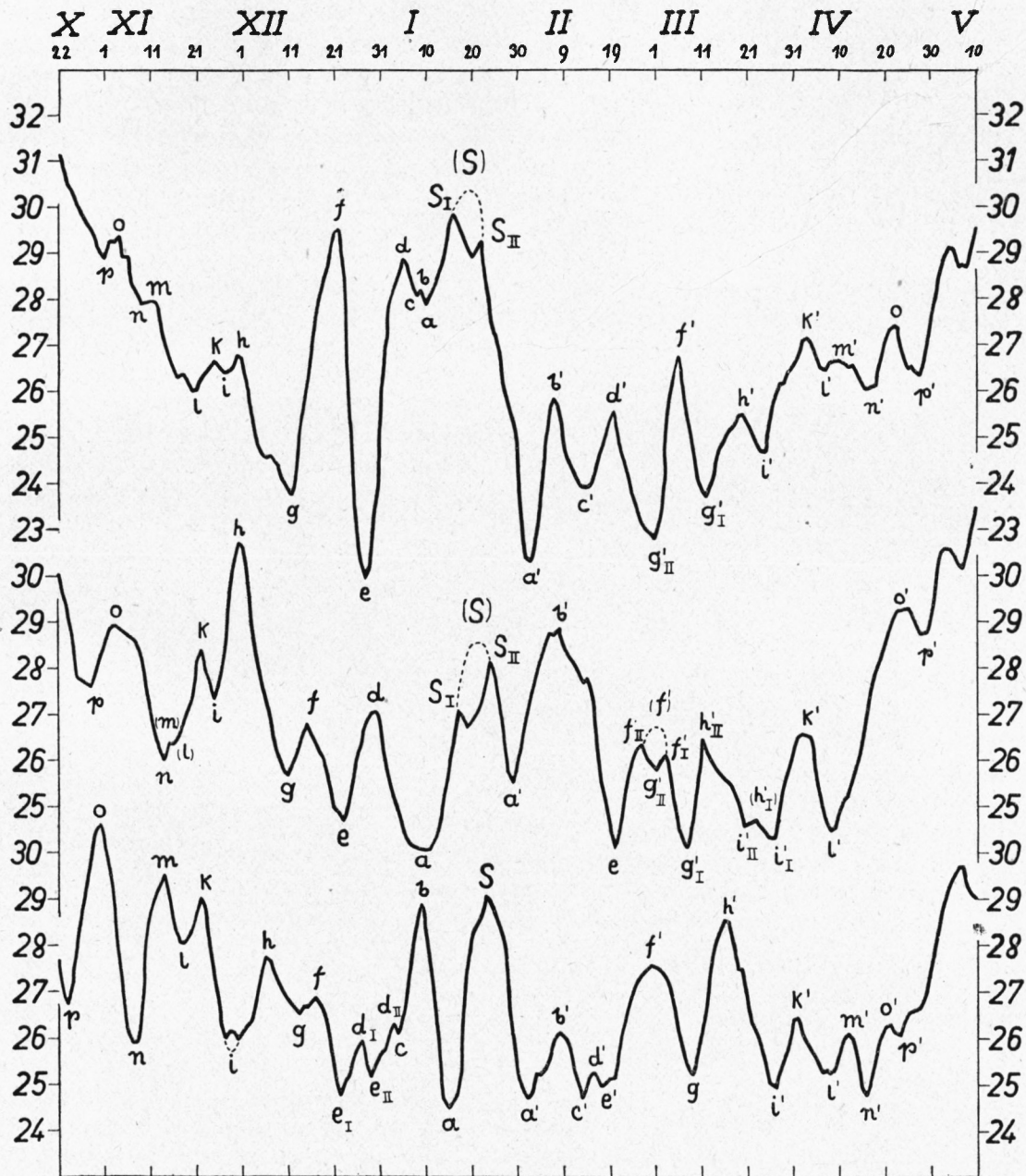
Bild 13. Verlauf des Luftdruckes auf der Zugspitze im Bereiche' des Winterspiegelungspunktes in übergreifenden Pentadenmitteln (500 + . . mm)
