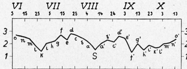
Bild 14 Mittlere Streuung des Eintrittsdatums der markanten Punkte im Sommer
