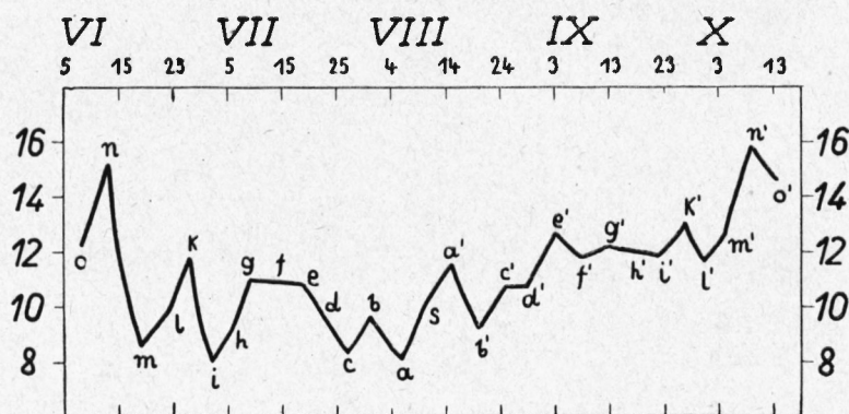
Bild 18. Mittlere Abweichungen des Luftdrucks in mm an den markanten Punkten der einzelnen Jahre im Sommerabschnitt
