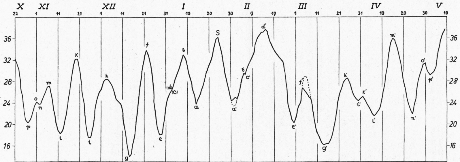
Bild 25 Gang des Luftdrucks auf der Zugspitze in übergreifenden Pentadenmitteln (500 + . . mm) im Winter 1933/34
