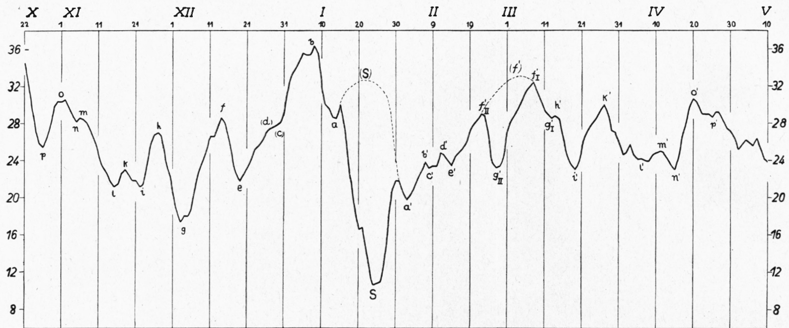
Bild 22. Gang des Luftdrucks auf der Zugspitze in übergreifenden Pentadenmitteln (500 + .. mm) im Winter 1909/10
