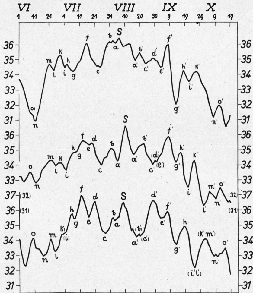
Bild 12. Verlauf des Luftdruckes auf der Zugspitze im Bereiche des Sommerspiegelungspunktes in übergreifenden Pentadenmitteln (500 + . . mm)
