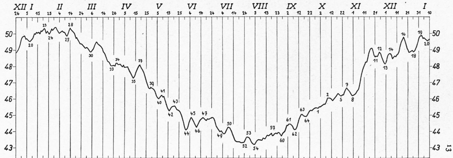
Bild 6. Mittlere Abweichungen der Druckdifferenz Hohenpeißenberg-Zugspitze für jeden Kalendertag in übergreifenden Pentadenmitteln (mm)
