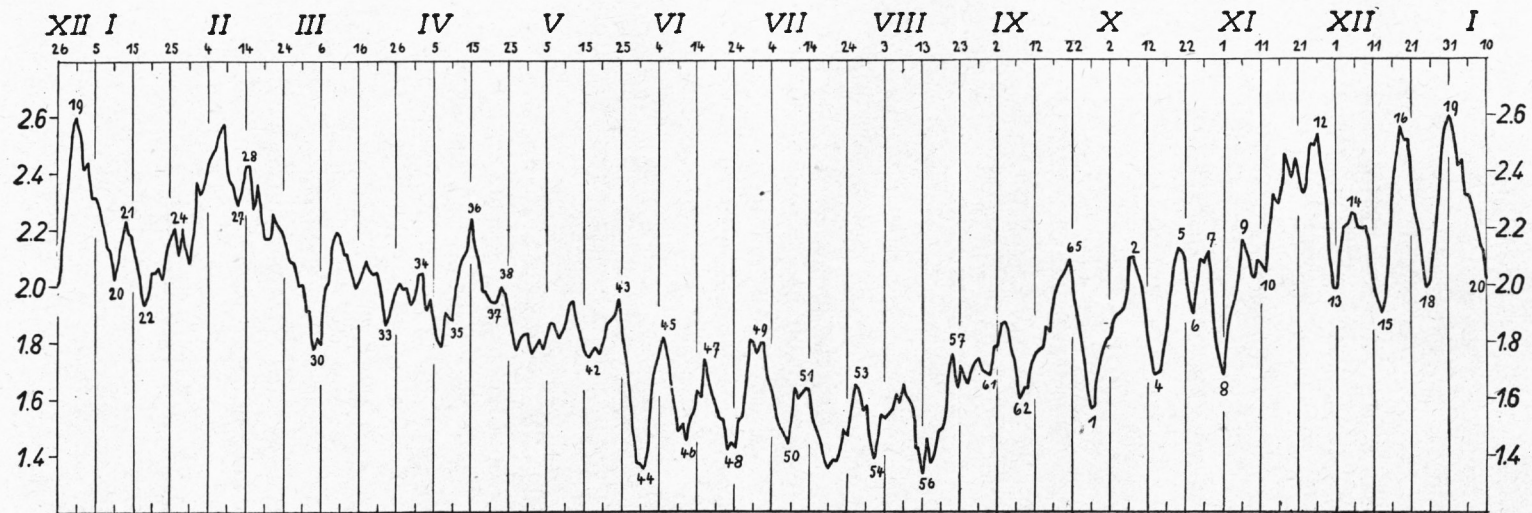
Bild 5. Jährlicher Gang der Druckdifferenz Hohenpeißenberg-Zugspitze in übergreifenden Pentadenmitteln (100 + . . mm) 1901-1930 für den Termin 21 Uhr
