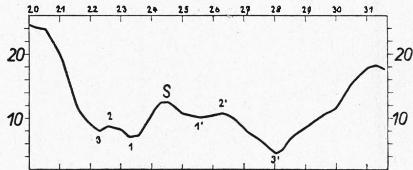
Bild 24 Verlauf des Luftdrucks vom 20. bis 31. Januar 1915, dargestellt durch die drei Terminbeobachtungen (500 + . . mm)
