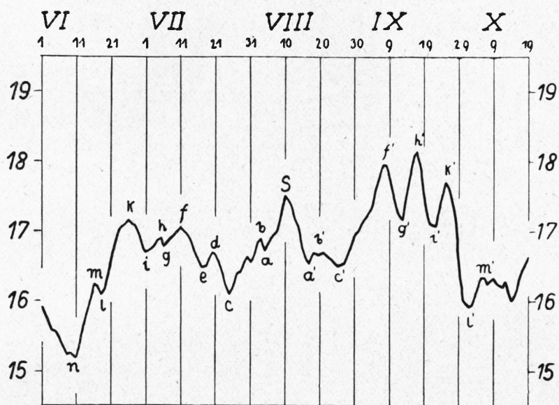
Bild 10 Verlauf des Luftdruckes in München (700 + . . mm) im Bereiche des Sommer- spiegelungspunktes in übergreifenden Pen- tadenmitteln
