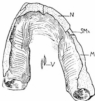
Fig. 5. Pachyrhines kaiseri nov. gen. nov. sp. Fundort wie Fig. 1. Querbruch durch die Schnauze vor den Alveolen der Caninen. Das vertikale Septum des „Vomer“ V ist weiter rückwärts, etwa in der Höhe des Diastema zwischen Caninen und erstem Postcaninen, durchgebrochen und zeigt hier deutlich, daß es aus zwei Lamellen besteht. — \frac{1}{2} nat. Gr.
