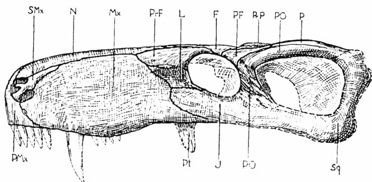
Fig. 1. Pachyrhinos kaiseri nov. gen. nov. sp. Karrooformation, unt. Beaufort-Schichten, Tapinocephalus-Zone (ob. Perm). Farm La-de-da bei Beaufort West, Kap-Provinz, Südafrika. — Rekonstruktion des Schädels. Seitenansicht. — \frac{1}{4} nat. Gr.
