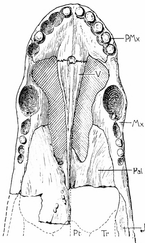
Fig. 4. Pachyrhinos kaiseri nov. gen. nov. sp. Fundort wie Fig. 1. Schädelunterseite, vorderer Teil. Halbschematisch. — \frac{1}{2} nat. Gr.
