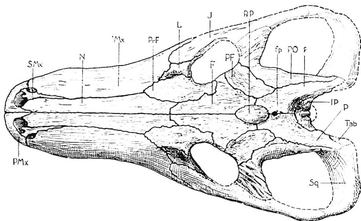
Fig. 2. Pachyrhinos kaiseri nov. gen. nov. sp. Fundort wie Fig. 1. Rekonstruktion des Schädels. Oberseite. — \frac{1}{4} nat. Gr.
