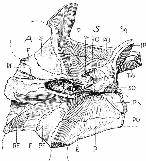
Fig. 3. Pachyrhinos kaiseri nov. gen. nov. sp. Fundort wie Fig. 1. Unterseite der rückwärtigen Partie des Schädeldaches, etwas verdrückt und daher nicht ganz symmetrisch erscheinend. — \frac{1}{2} nat. Gr.
