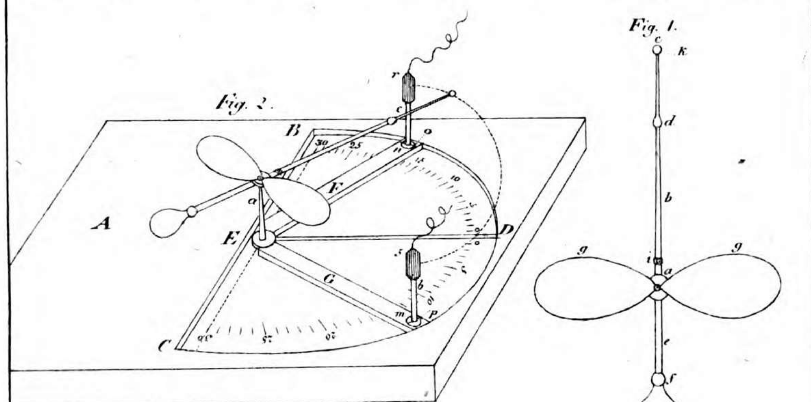
Fig. 1. Oscillations Libelle für Horizontal-Schwingungen. im \frac{1}{4} Theil ihrer wahren Grösse.
