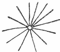
die Büschelpunkte
