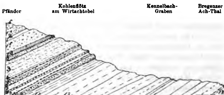
I. Profil durch die Molasse-schichten von dem Bregenzer-Achthale in nördlicher Richtung bis zum Pfänder.
