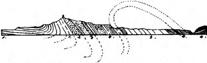
III. Profil durch die oberoligozänen und miocänen Schichten am hohen Poissenberg (1:50000). 1) Obere Süßwassermolasse; 2) Conglomerat derselben; 3) Zwischenregion mit einer Lage der Ostrea crassissima ; 4) Cyrenenmergel mit Pechkohlenflötzen; 5) ältere brackische Molasse.
