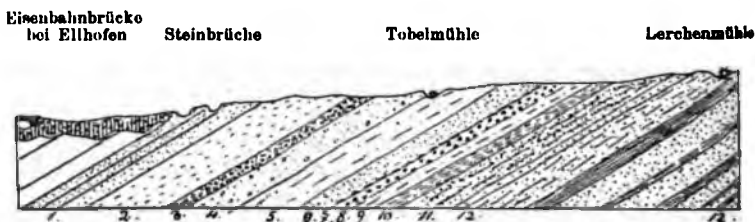
II. Profil durch den Ellhofener Tobel bei Simmerberg (nach der Linie des Einfallens reduziert) 1:50000.
