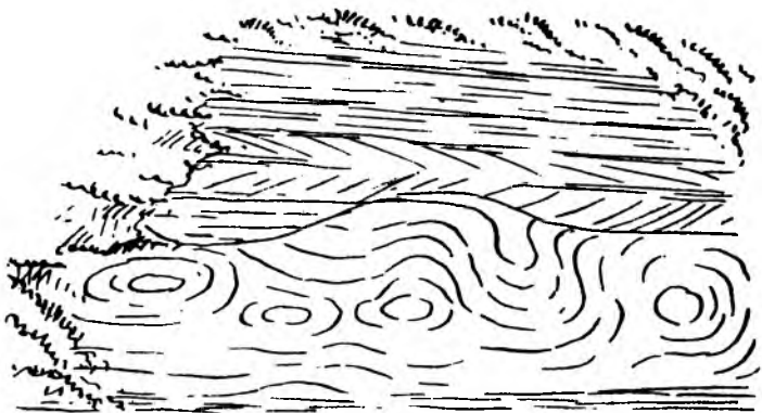
Schichtenbiegungen in einer Sandgrube bei Ottnang.
