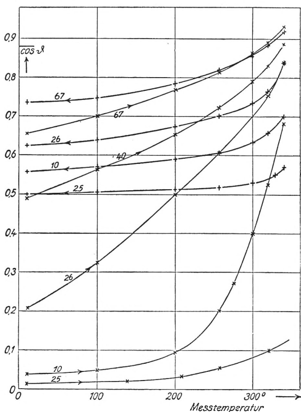
Abb. 6. Thermische Idealisierungskurve von hartem Nickel ( H_i = 25,5 Oe) Parameter: H_i in Oe
