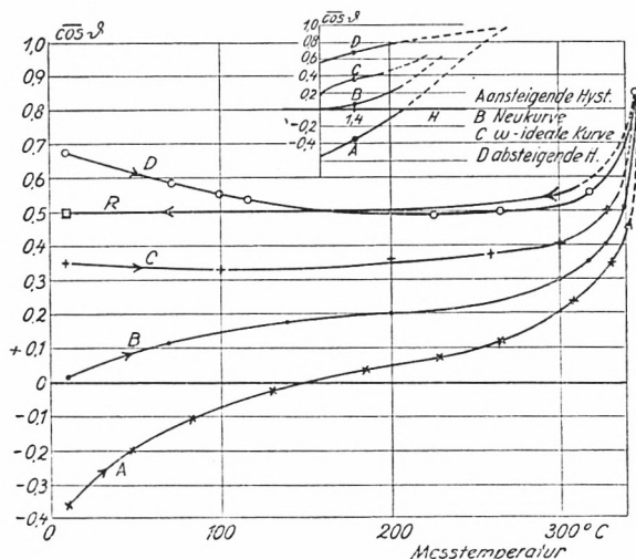
Abb. 4. Thermische Idealisierungskurven bei verschiedenen Ausgangszuständen (siehe Nebenfigur) in H_i = 1,4 Oe
