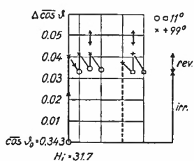
Abb. 15. Änderung von \overline{\cos \vartheta} bei mehrfachem Temperaturwechsel. ○ 11^\circ C (Ausgang) × 99^\circ C; + 99^\circ C (Ausgang) □ 11^\circ C hartes Nickel
