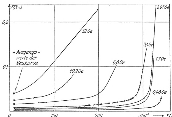
Abb. 8. Einsatztemperatur der irreversiblen Prozesse ( \overline{\cos \Theta} -Werte) bei verschiedenen Feldstärken (Parameter: H_i in Oe)
