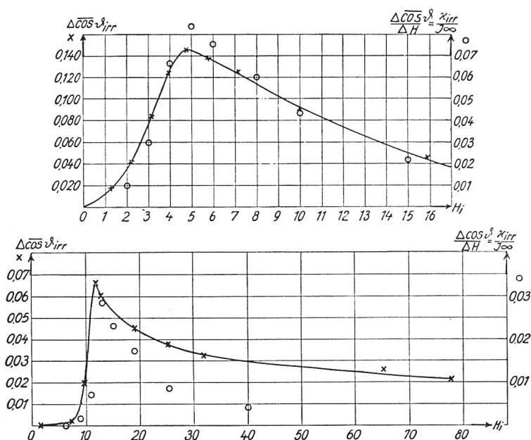
Abb. 17. Die irreversible \overline{\cos \vartheta} -Änderung beim Wechsel 11^\circ - 99^\circ - 11^\circ (zum Vergleich: die reduzierte irreversible Suszeptibilität bei 11^\circ C bei gleichen Feldstärken)
