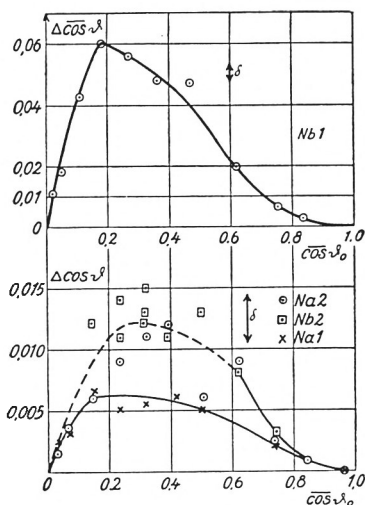
Abb. 18. Die Beträge der irreversiblen Nachidealisierung.
