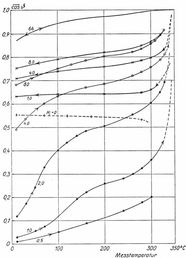
Abb. 2. Thermische Idealisierungskurven: \overline{\cos \theta} = \text{Werte} . Änderung von \overline{\cos \theta} bei steigender und fallender Temperatur. Parameter: H_i in Oersted.
