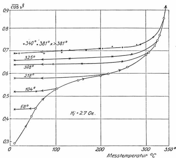
Abb. 11. Partielle thermische Idealisierung in konstantem H_i . Parameter der Rückgangskurven: maximale Erhitzungstemperatur
