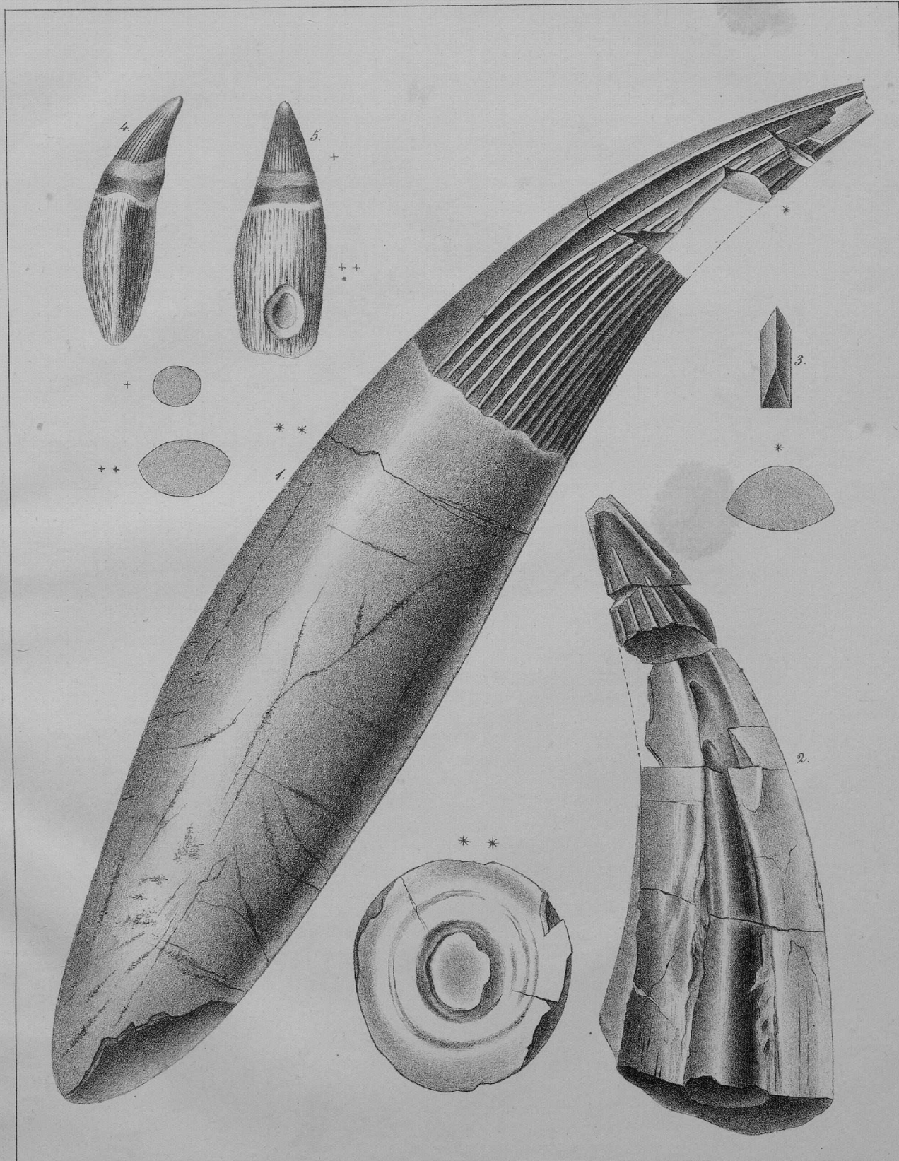
Fig. 1_3. Pliosaurus giganteus . Fig. 4_5. Ichthyosaurus posthumus .
