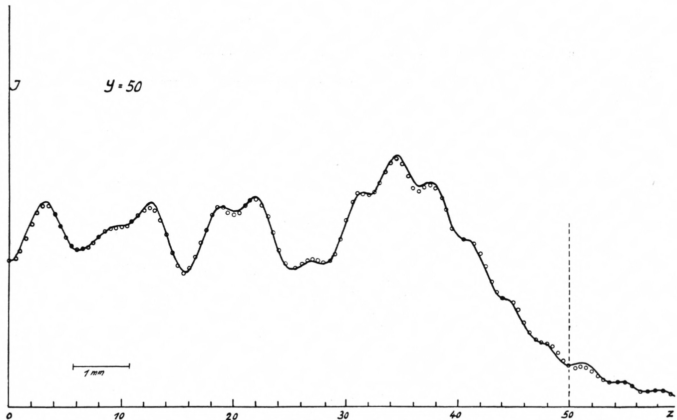
Abb. 15 Theoretische (mit e = 0,5 ) und gemessene Beugungsfigur. Versuchsbedingungen: a = 58,1 mm b = 1098,5 mm d = 0,973 mm \lambda = 5461 \text{ \AA} Bel. Spalt etwa 7\mu Aufn. Spalt etwa 50\mu
