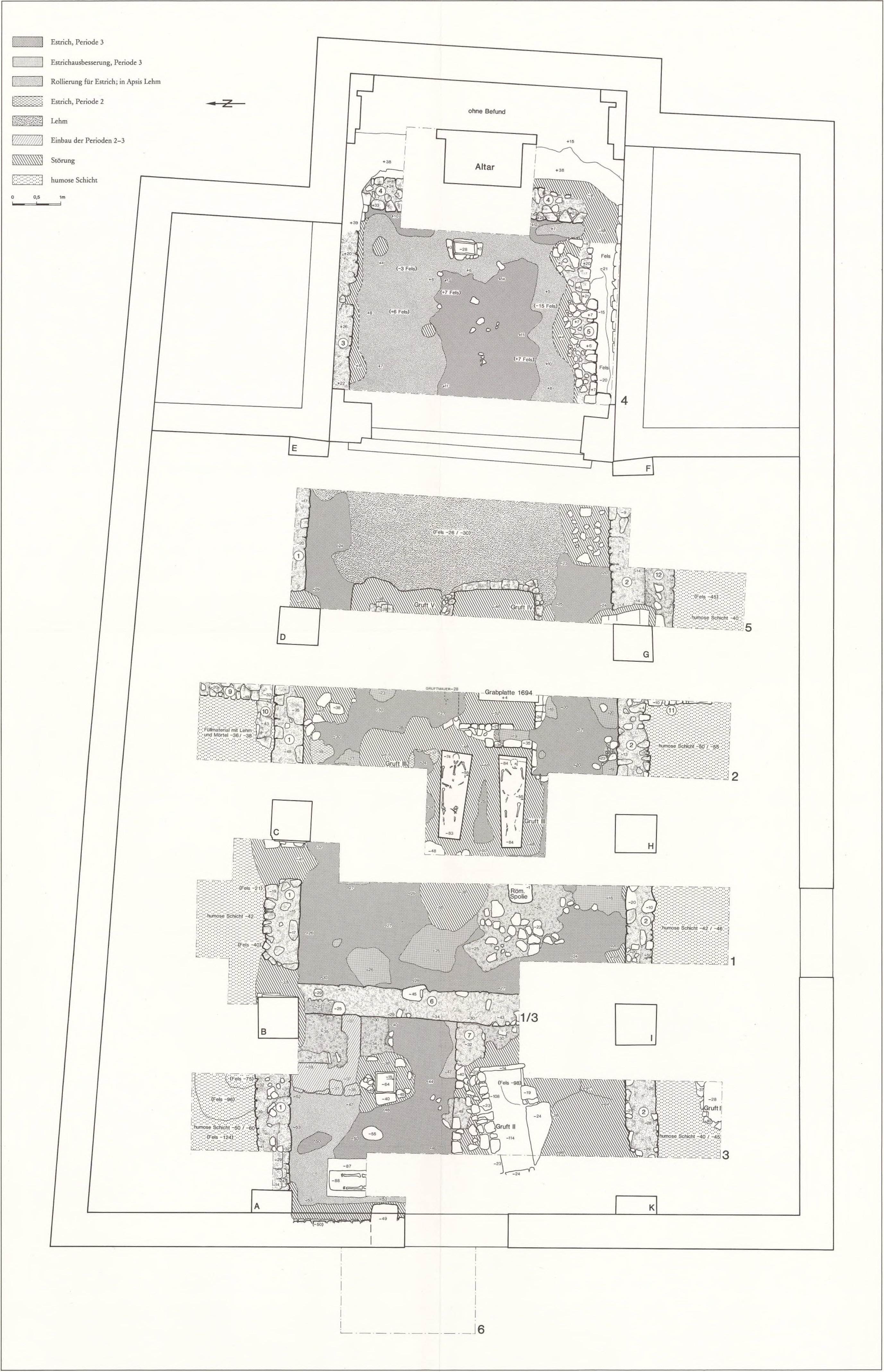
Invillino, Colle Santino, S. Maria Maddalena. Gesamtplan von Bau I, Periode 3. M. 1:50.
