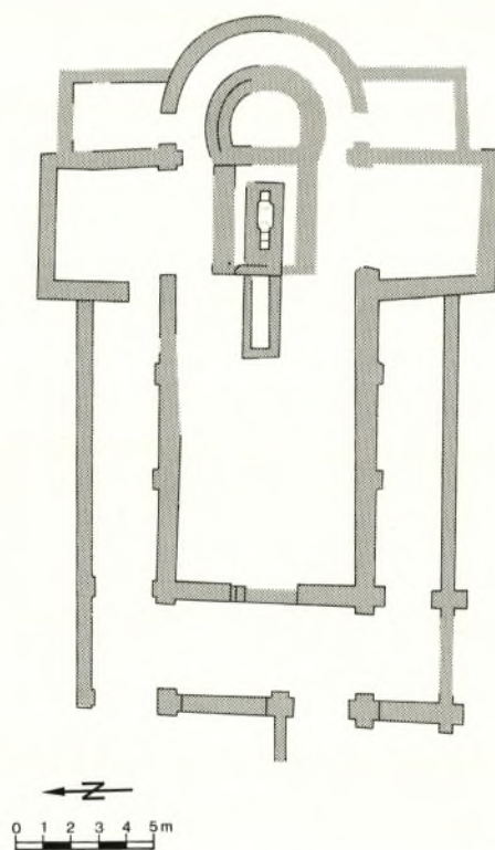
Abb. 16. Sabiona-Säben (vgl. Anm. 53). M. 1:300.
